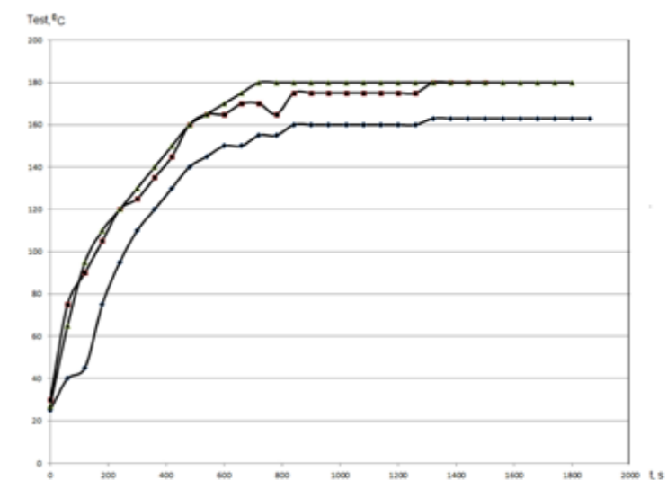
Figura 3. Gráficas de la temperatura del esterilizador en función del tiempo.
